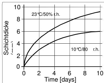
Diagramm 1: Durchhärtengeschwindigkeit für Sikaflex®-290i DC
